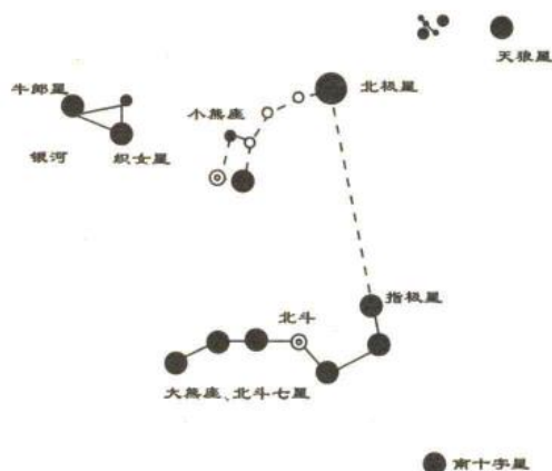
判断方位之北极星星象图
