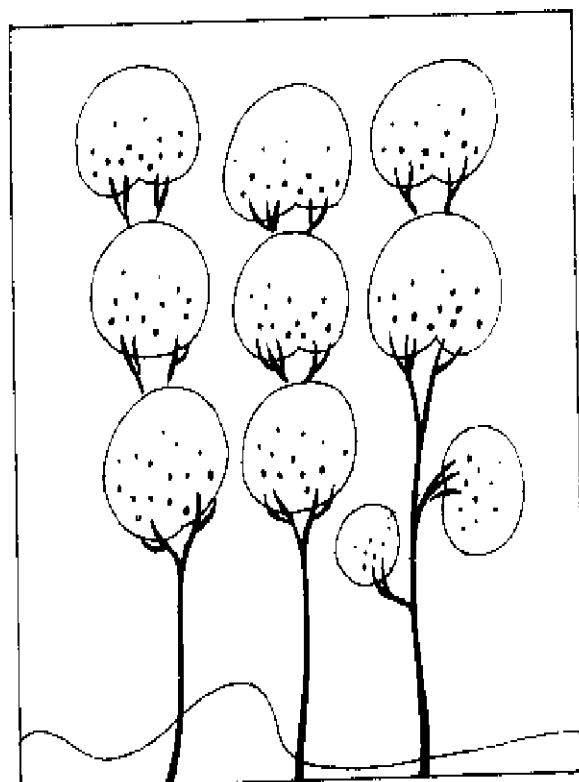
树 形
