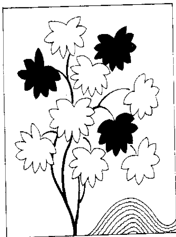
树 形
