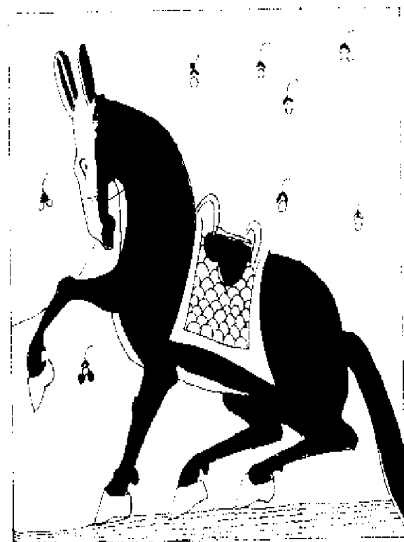
动物
