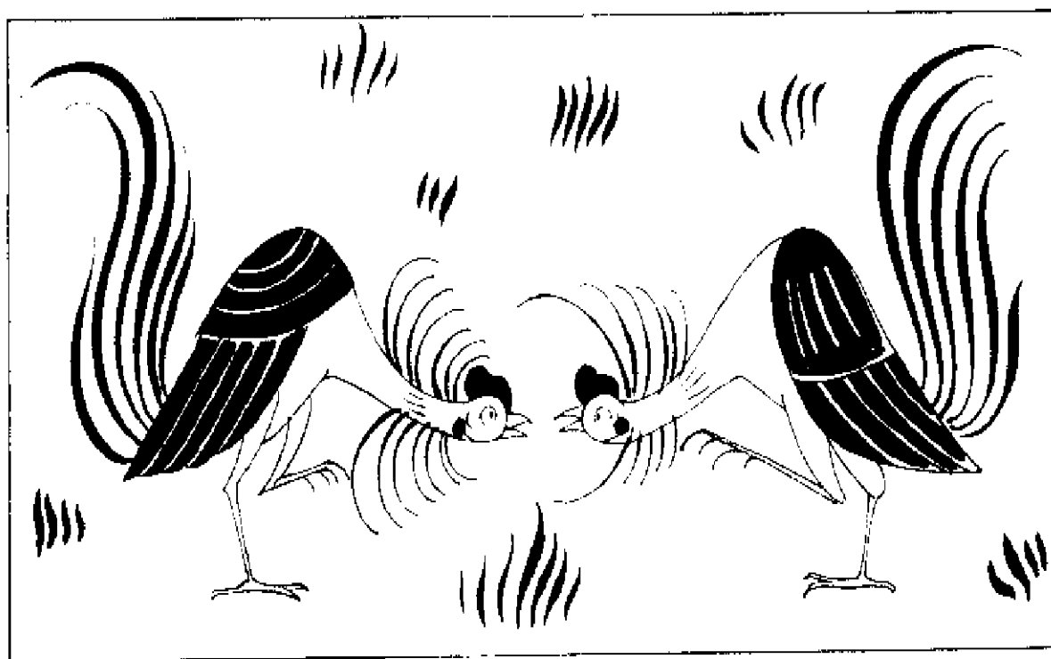
幼 物
