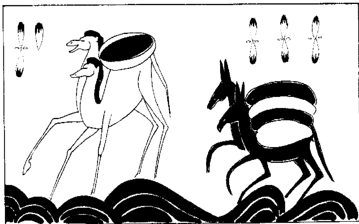
动 物
