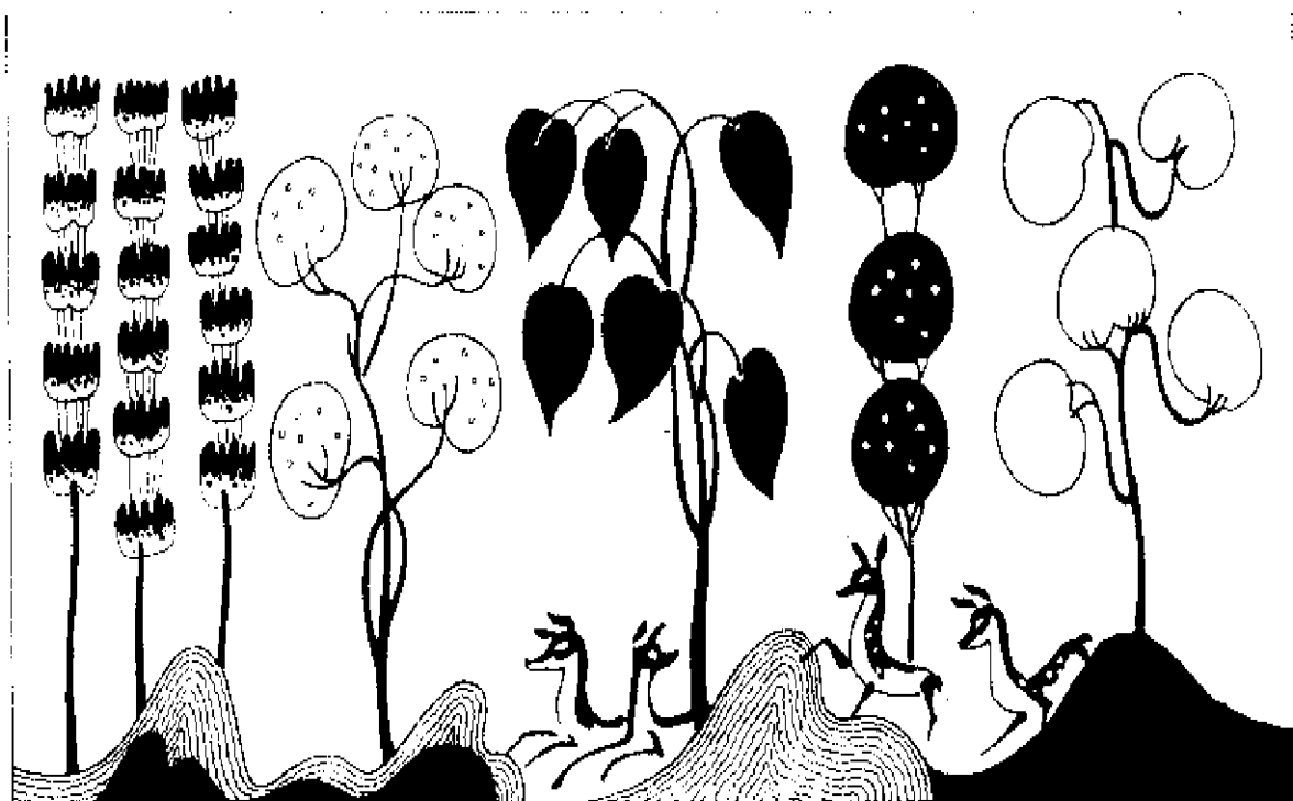
树 形
