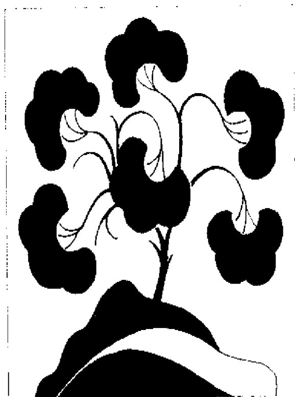
樹 形
