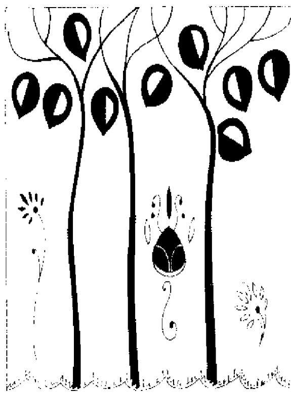
树 形
