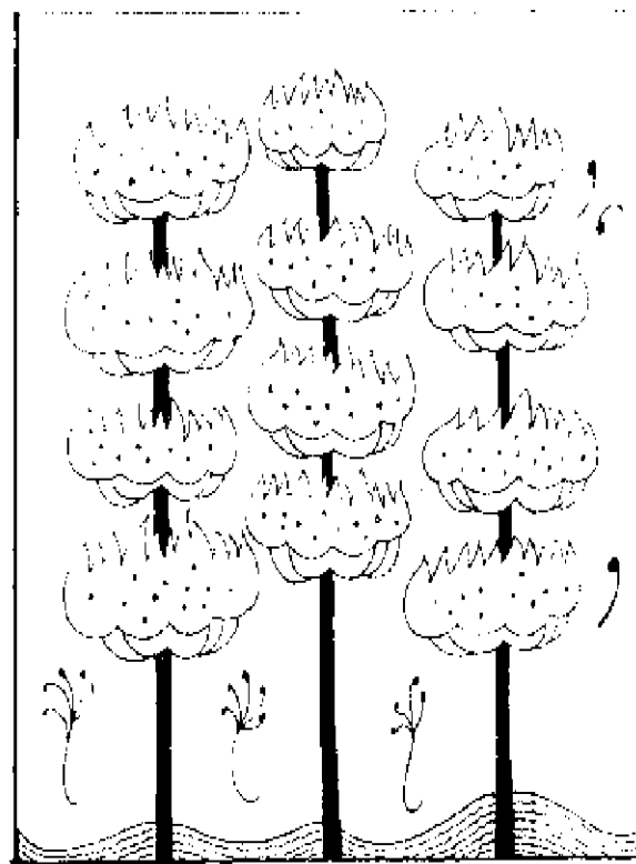
树 形
